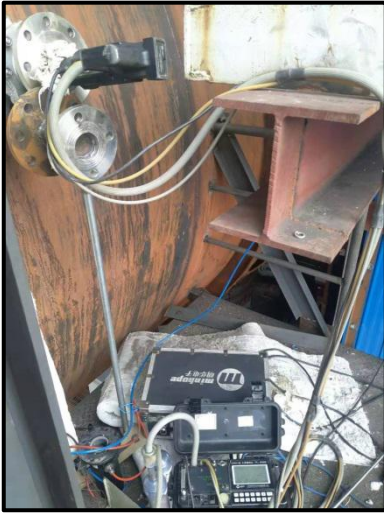
5#、6#焦炉处理设施前废气采样
