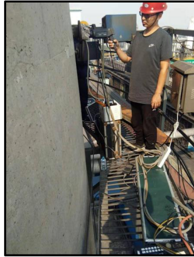
5#、6#焦炉处理设施后废气采样
